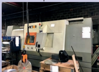
Tour CNC VICTOR VTURN 46 2 axes De 2006 Dia 730 x 1700 mm CNC Fanuc 21 T
