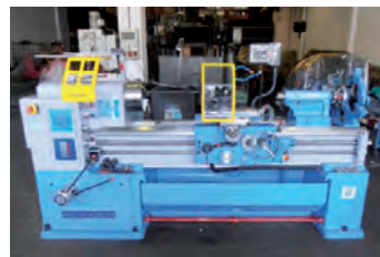
AV Tour parallèle CAZENEUVE Type HB 575 x 1500 - Reconstitue Distance entre pointe : 1500 mm Hauteur de pointe : 250 mm - ø admis au-dessus du banc : 575 mm - ø admis au-dessus du chariot : 340 mm - Alésage broche : 52 Conicité de la contre pointe : CM5 Course maxi du chariot transversal : 400 mm - 18 vitesses de broche : 25 à 2000 tr/min - Puissance moteur de broche : 8,8 kw Dimensions machine : 2400 x 1180 x 1350 - Protection mandrin Tél : 06 07 68 86 74
